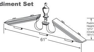
PEDIMENTST Pediment Set
